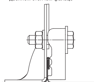
Применение кронштейна на двойном стоячем фальце
