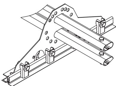
Кронштейн со скобами
